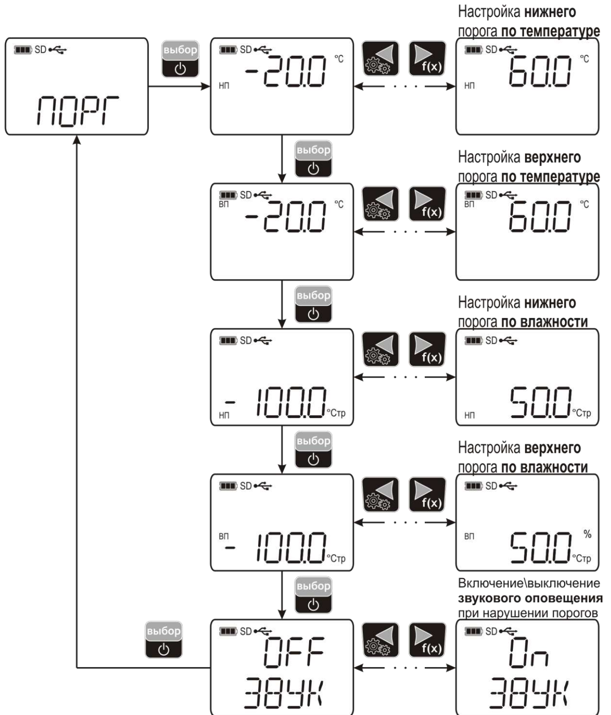
Рисунок 5.3 Установка порогов
